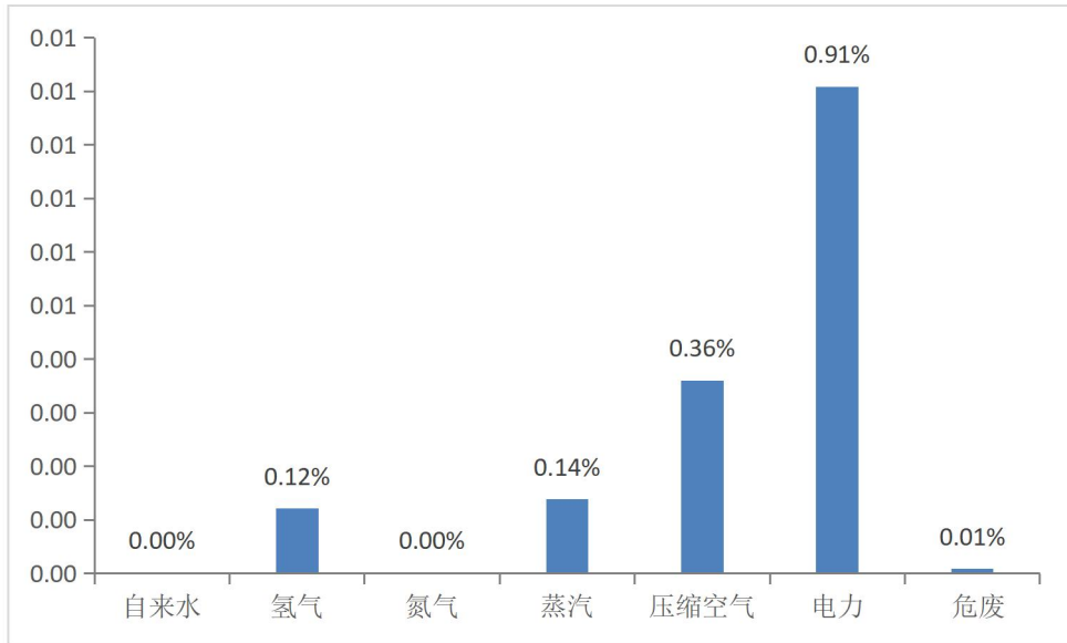
图 9 焦磷酸二氢二钠生产阶段各清单过程RU-F贡献柱状图
