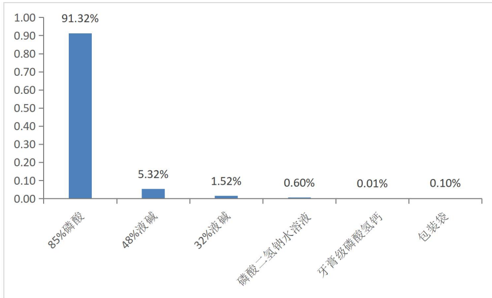
图 11 焦磷酸二氢二钠原材料获取和加工阶段各清单过程RU-M贡献柱状图
