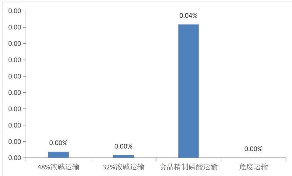
图 8 焦磷酸二氢二钠原材料运输阶段各清单过程RU-F贡献柱状图
