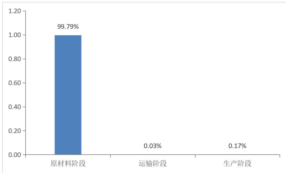
图 18 焦磷酸二氢二钠生产阶段各清单过程HT贡献柱状图
