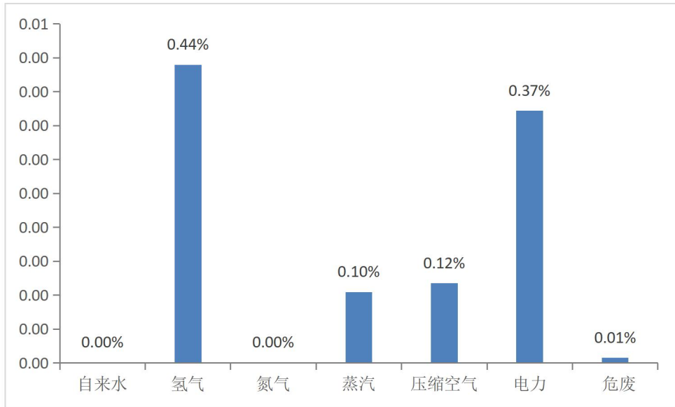
图 13 焦磷酸二氢二钠生产阶段各清单过程RU-M贡献柱状图
