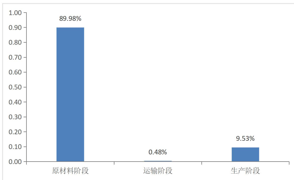
图 2 焦磷酸二氢二钠各阶段清单过程GWP贡献柱状图
