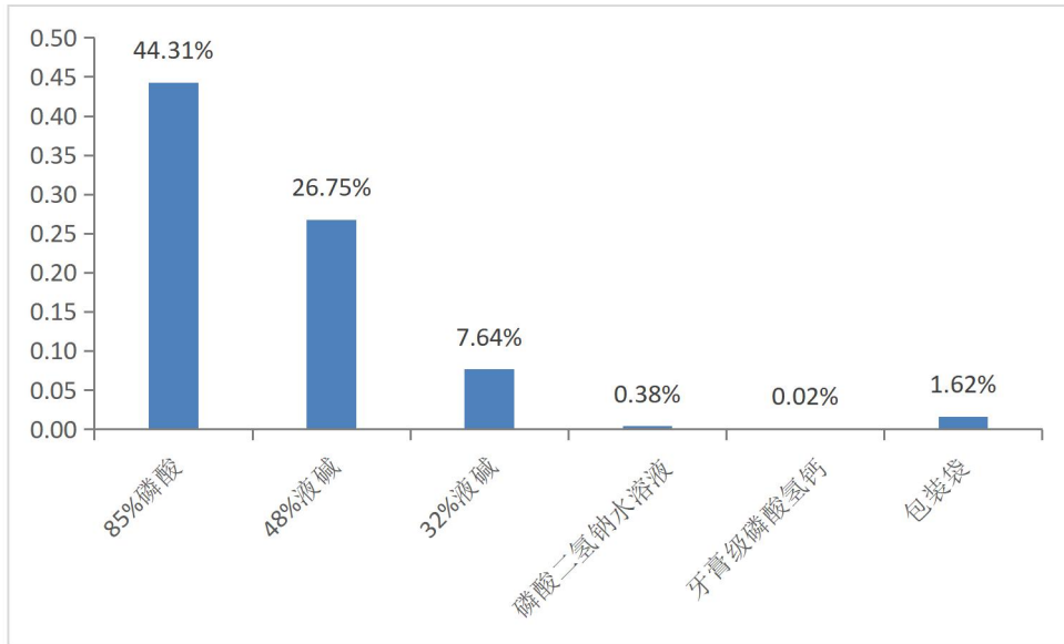
图 15 焦磷酸二氢二钠原材料获取和加工阶段各清单过程EF贡献柱状图
