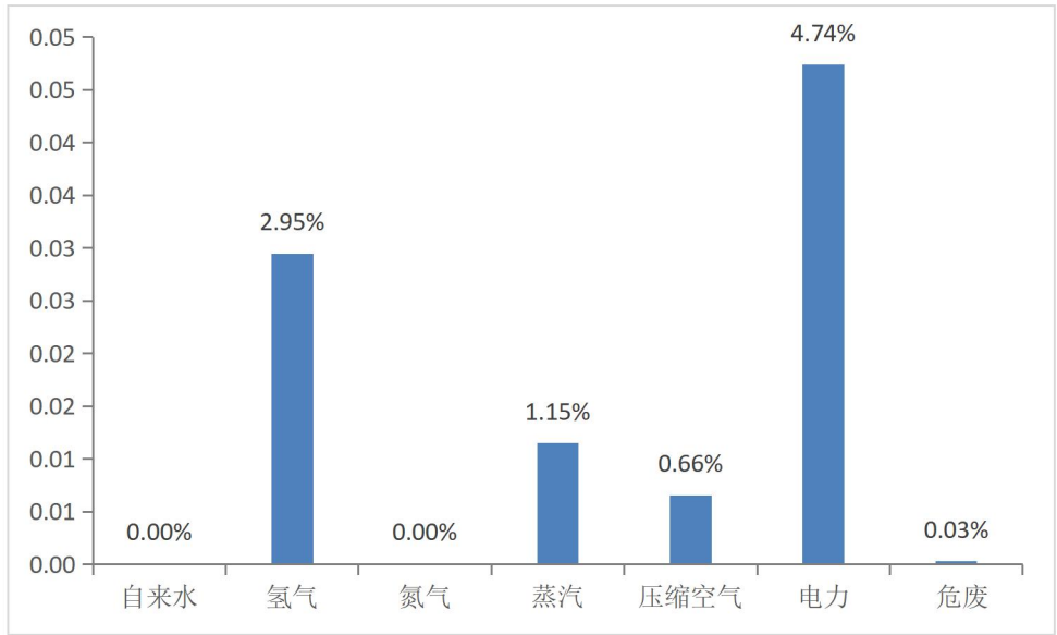
图 5 焦磷酸二氢二钠生产阶段各清单过程GWP贡献柱状图
