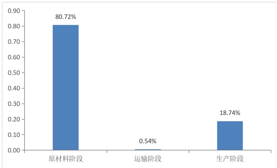
图 14 焦磷酸二氢二钠生产阶段各清单过程EF贡献柱状图
