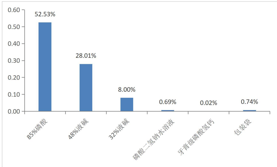
图 3 焦磷酸二氢二钠原材料获取和加工阶段各清单过程GWP贡献柱状图
