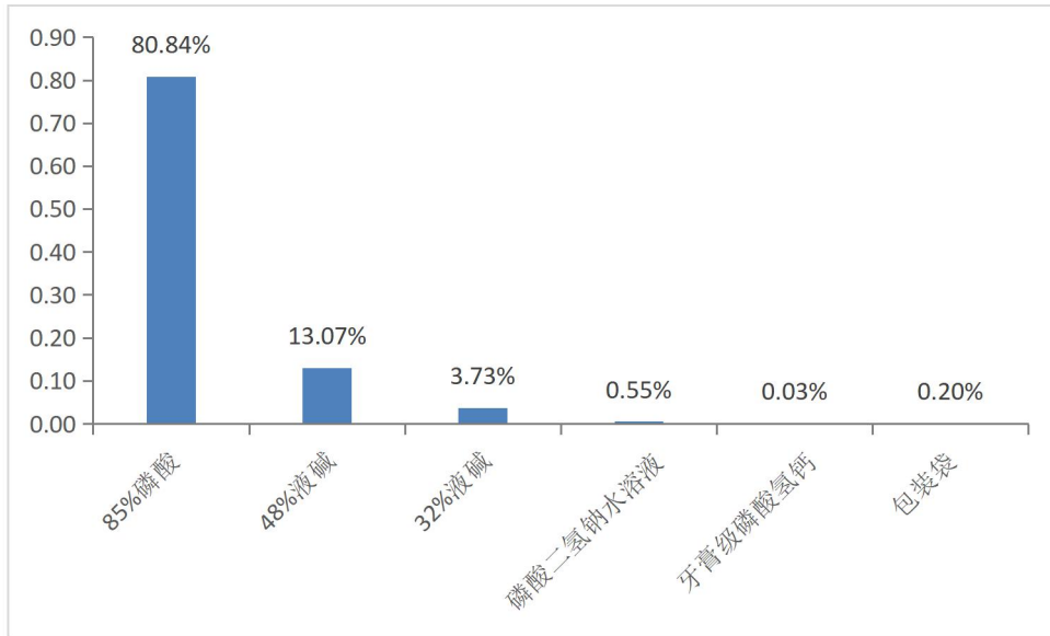
图 7 焦磷酸二氢二钠原材料获取和加工阶段各清单过程RU-F贡献柱状图
