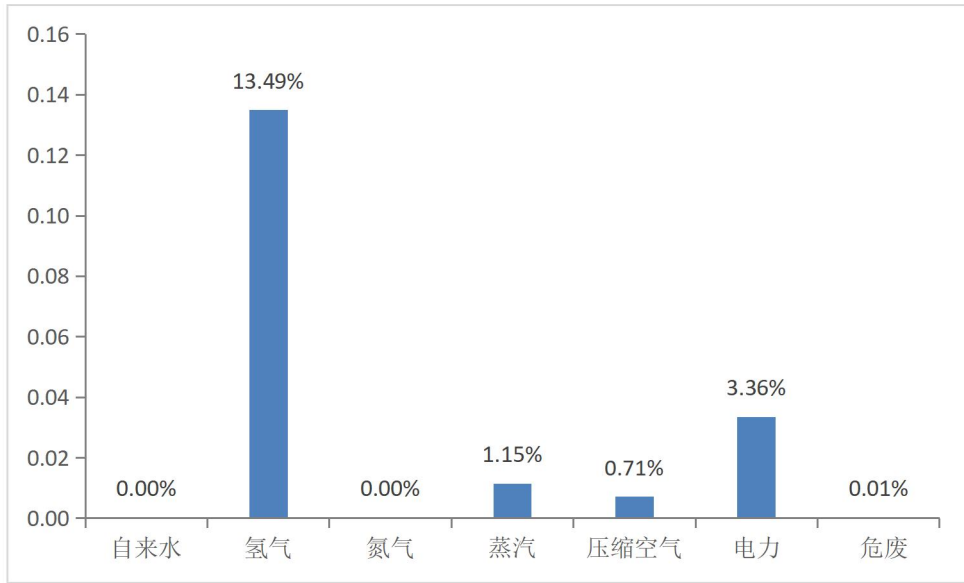
图 17 焦磷酸二氢二钠生产阶段各清单过程EF贡献柱状图
